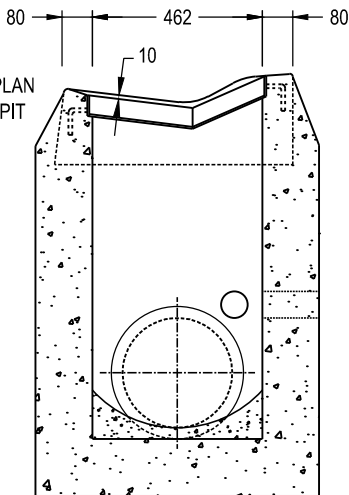
ELEVATION
