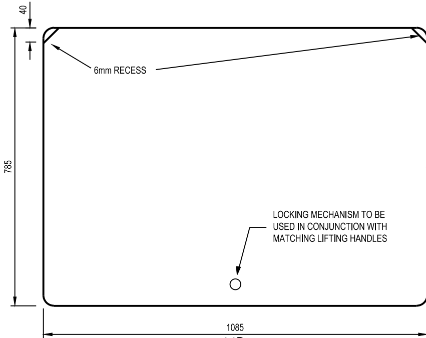
LID SCALE 1:10
