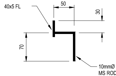
SECTION A-A SCALE 1:5
